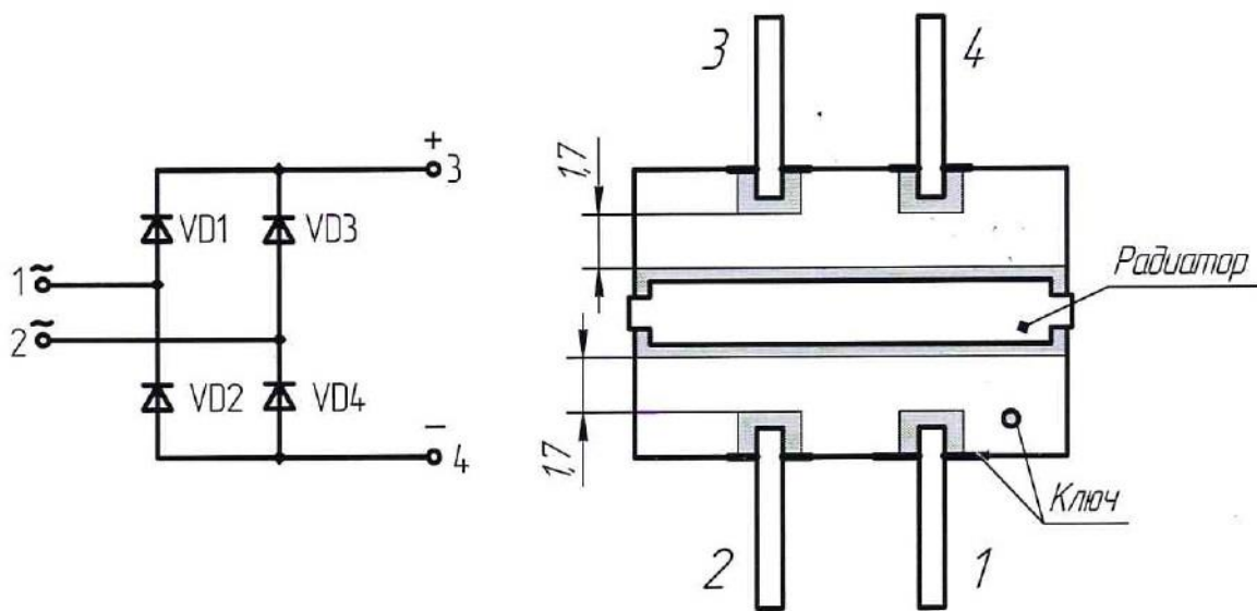
Рисунок 2 – Габаритный чертеж КТ-108-1 (ДФЛК.435711.006ГЧ)
