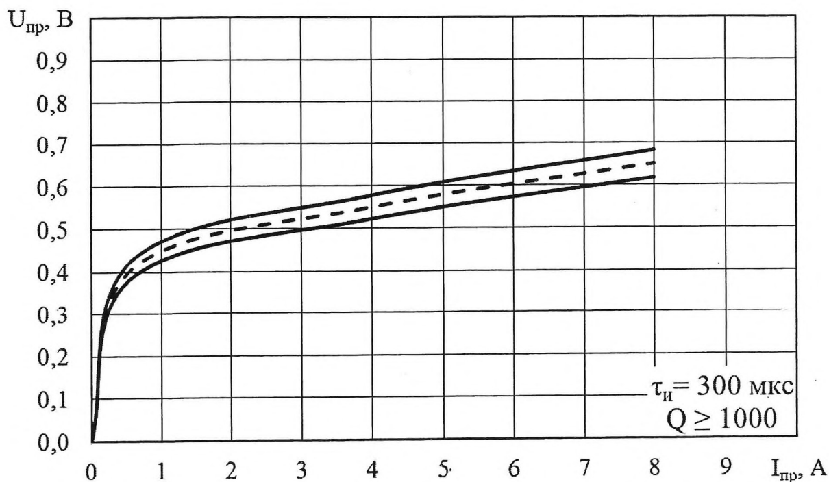
Рисунок Ж.1 – Область изменения прямого напряжения в зависимости от прямого тока при температуре корпуса t_{кор} = (-60 \pm 3) ^\circ\text{C} диода сборки КДШ161АС9
